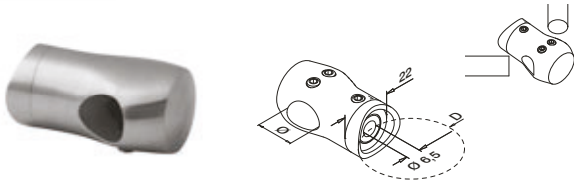
MOD 0839 - Ø 12 mm
