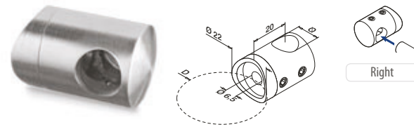
MOD 0833 - Ø 12 mm
