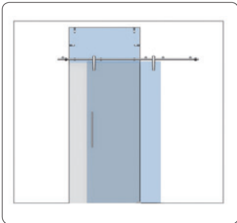
Typ 8 einflügelig, Anschluss Glas-Wand, Oberlicht
